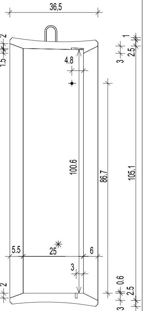
Schnitt A-A
