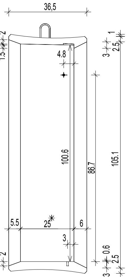
Schnitt A-A
