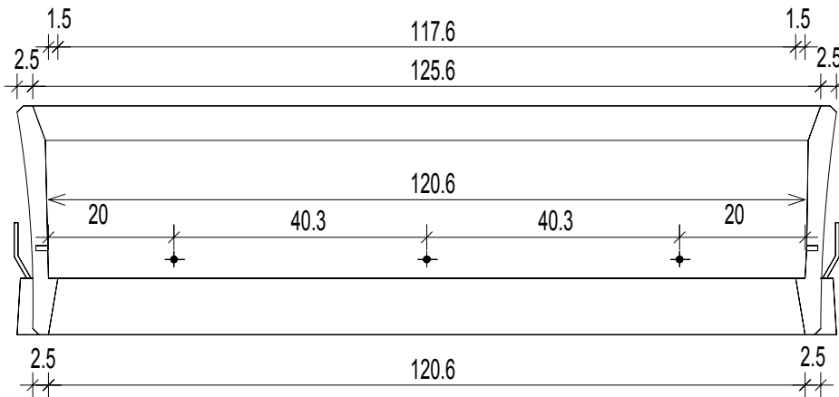
Schnitt B-B
