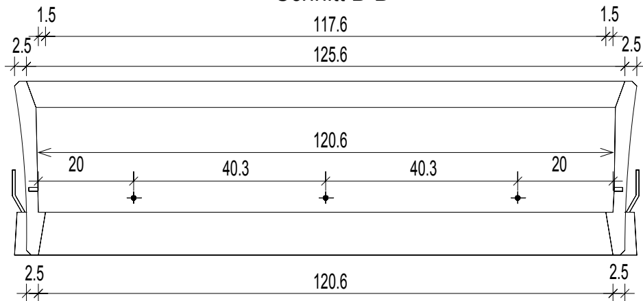
Schnitt B-B
